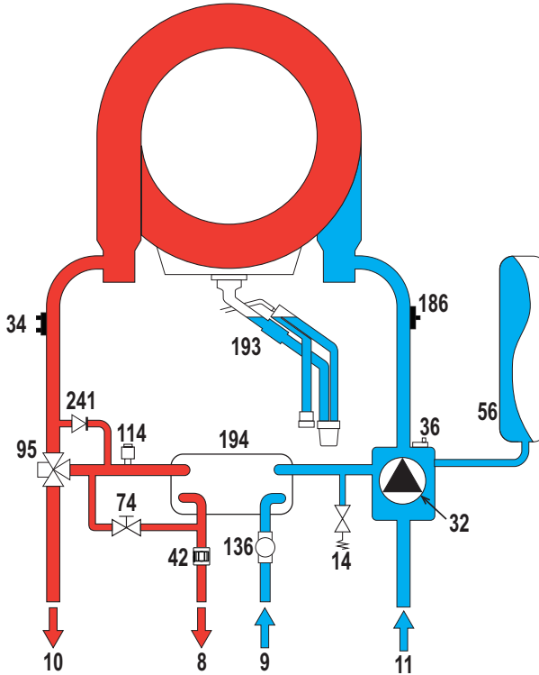
fig. 58- Circuitul hidraulic
