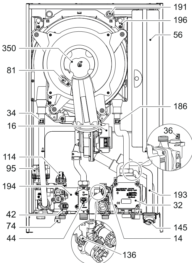
εικ. 57- Γενική όψη
