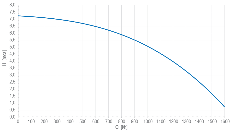
εικ. 59- Διαθέσιμο υπολειπόμενο μανομετρικό ύψος στην εγκατάσταση
