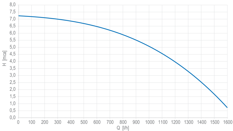
fig. 59- Înălțime de pompare reziduală disponibilă în instalație
