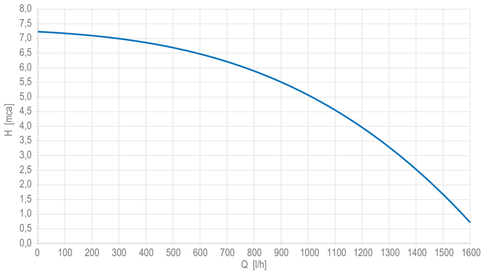
fig. 59- Carga hidrostática residual disponible en la instalación
