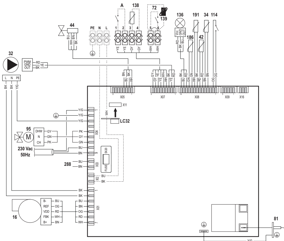
fig. 60 - Esquema eléctrico
