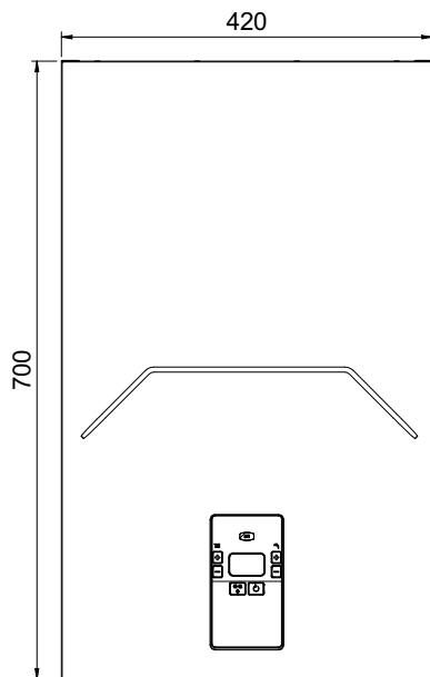
εικ. 49- Μπροστινή όψη
