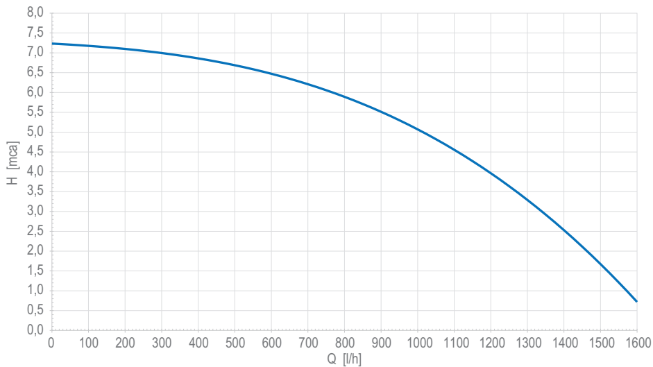
wygląd 59- Wysokość podnoszenia dostępna dla układu
