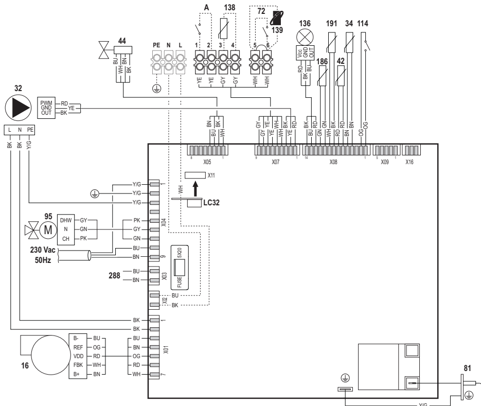
fig. 60- Wiring diagram
