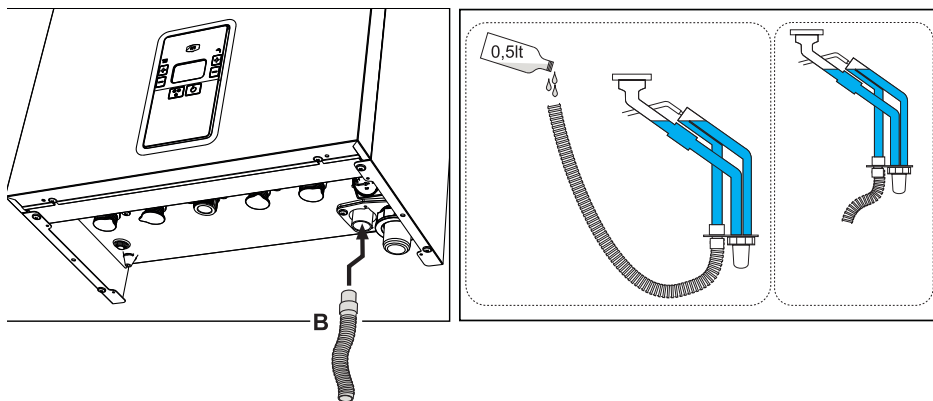
fig. 44- Conexión de la descarga de condensado
