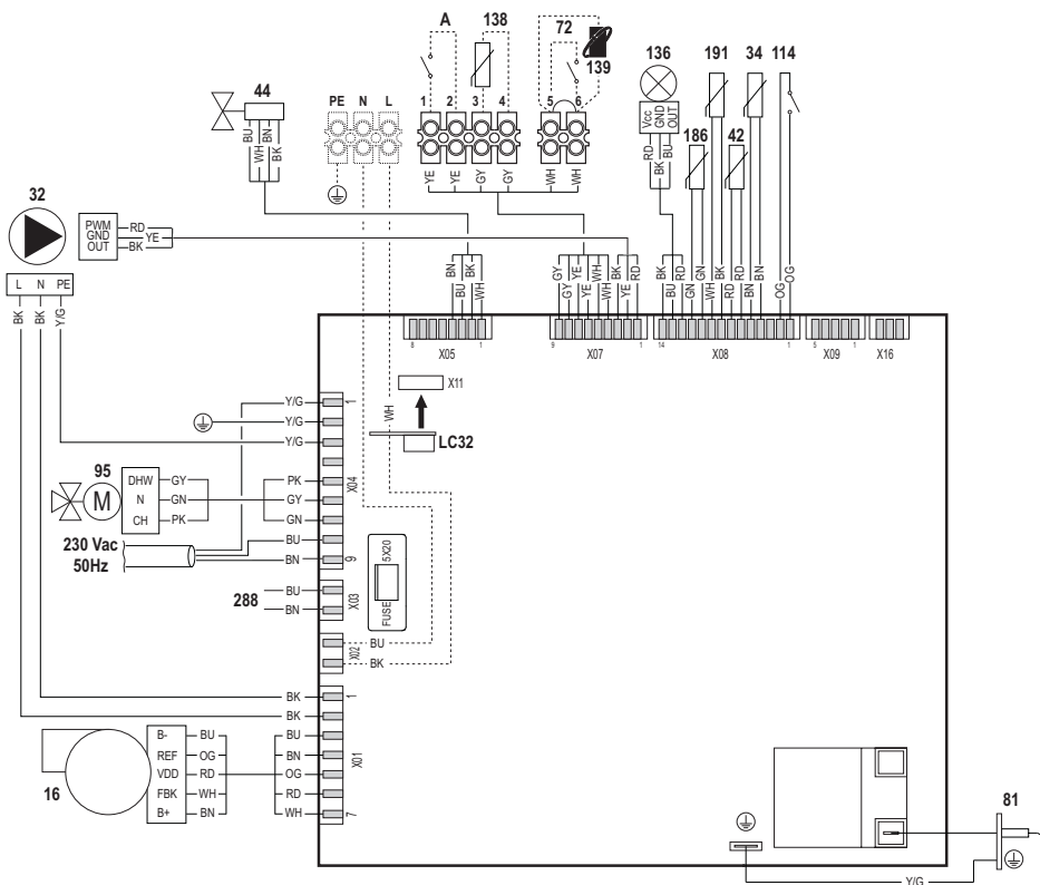
fig. 60- Schema electrică
