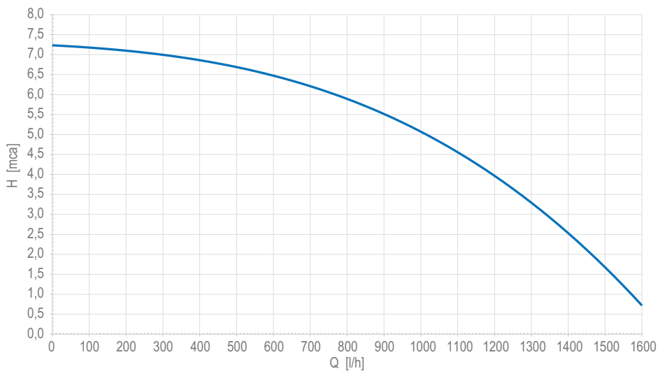
fig. 59 - Prevalenza residua disponibile all'impianto
