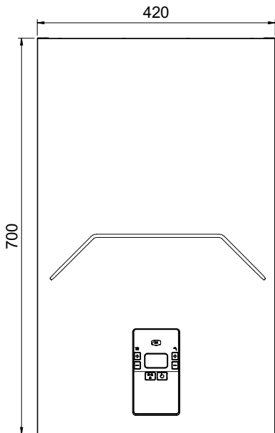
wygląd 53- Widok z przodu
