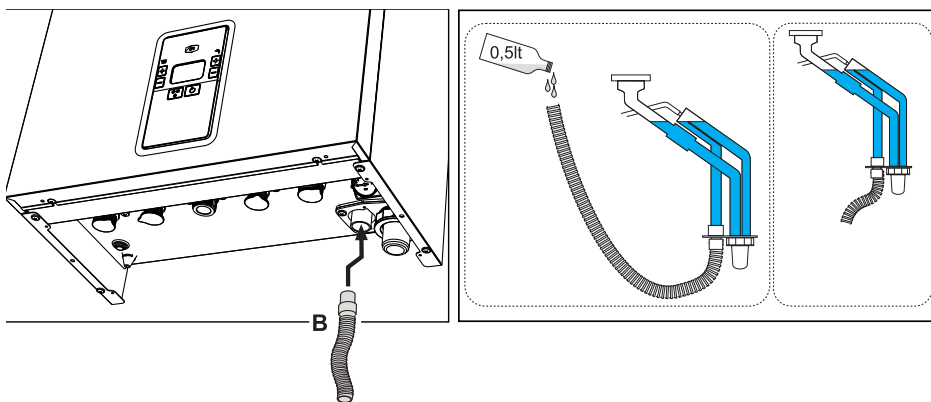
εικ. 44- Σύνδεση εξαγωγής συμπυκνώματος
